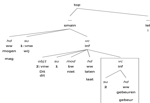
Figure 2. The Alpino dependency tree for the sentence “Dit mogen wij niet laten gebeuren! (En: We cannot let this happen! )”
